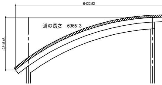
A - A' 断面詳細図 S=1:20
