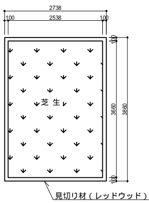
平面図
