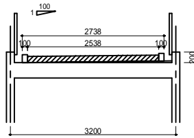
断面図
