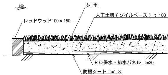
B - B' 断面詳細図 S=1:20
